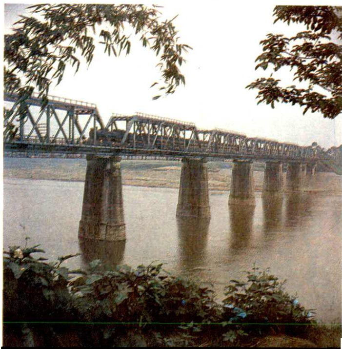
成渝铁路花江大桥
