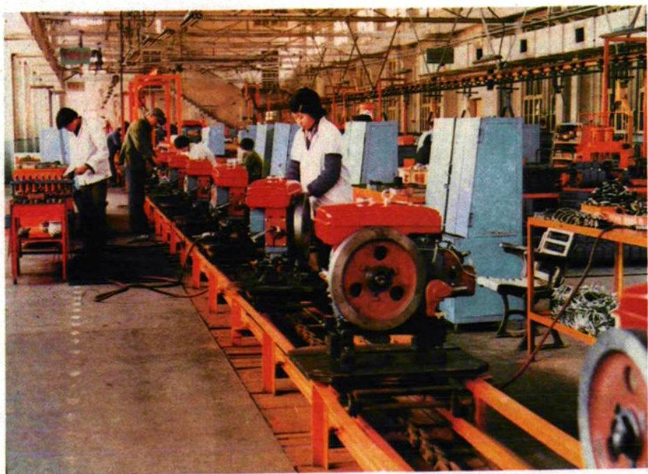
华丰机器厂的195 柴油机装配线
