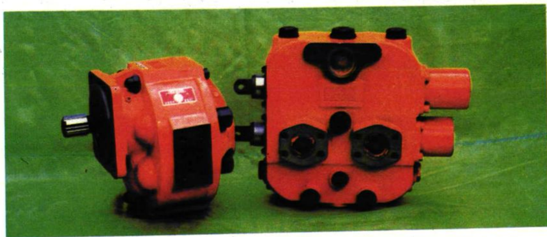
青州液压元件厂等单位研制的CBZ 4 高压大排量齿轮油泵(左)及DF型整体式多路阀(右)分获国家发明三等奖与省科技成果二等奖
