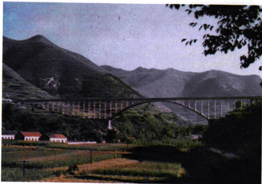
益都县水利局等单位用无支架缆索吊装技术建成的张庄百米跨双曲拱渡槽获1980年省科技成果三等奖
