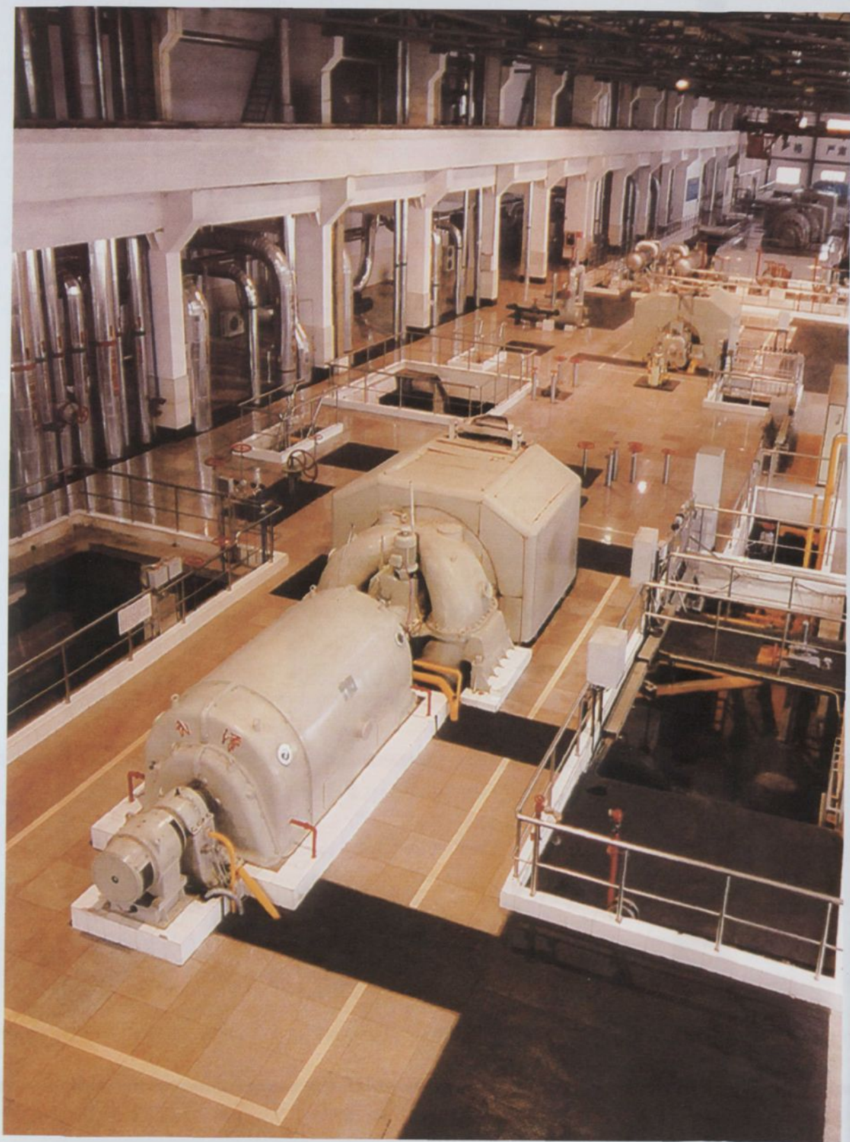
通辽热电厂汽机厂房
