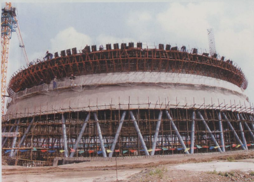
通辽热电厂六期工程水塔施工
