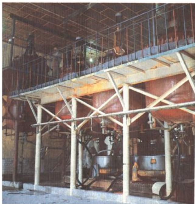
化工五厂草酸生产线
