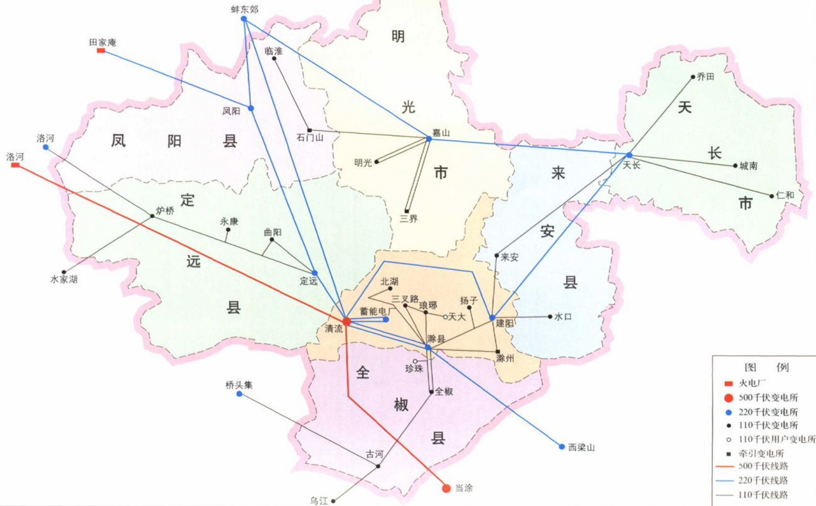
2005年度滁州电网地理接线示意图
