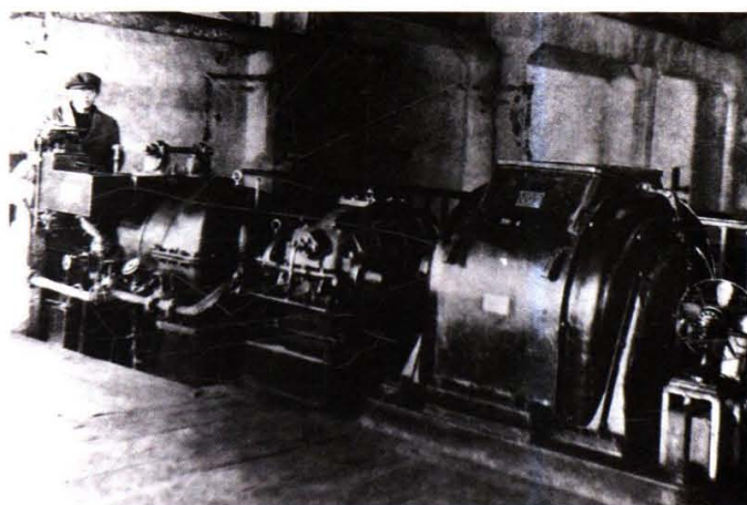
1942年投产的兰州电厂黄河沿发电所 500 千瓦发电机组
