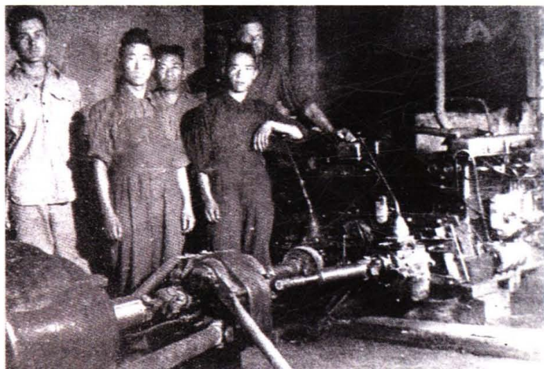
1945 年山丹培黎工艺学校 60 千瓦柴油发电机组
