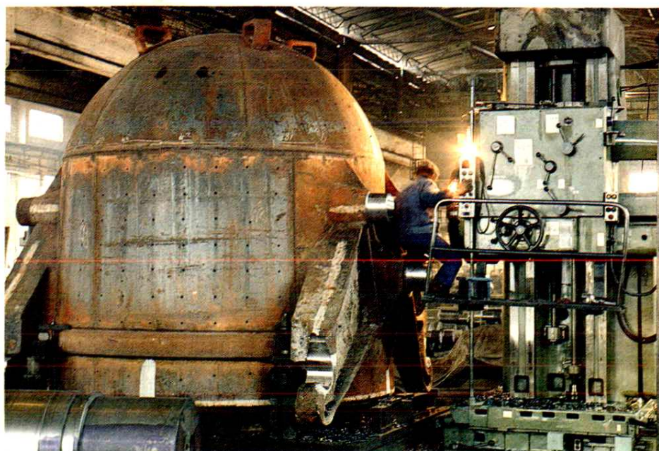
60吨铁水罐在 \Phi 160 镗床上加工
