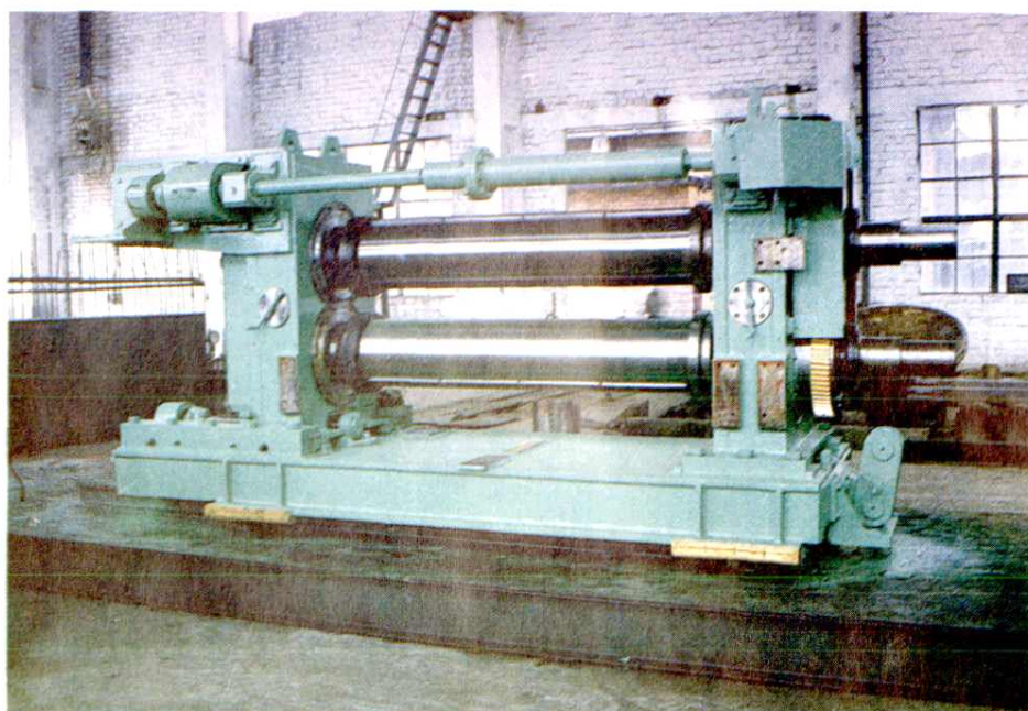
一米七轧机——纵剪机
