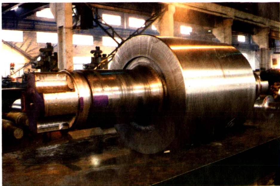
大中型球墨无限冷硬铸铁轧辊
