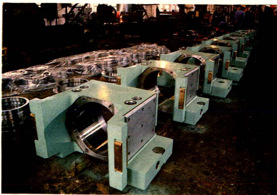
武钢一米七轧机轴承座
