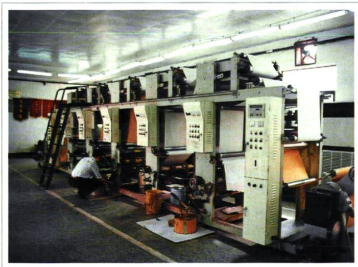
▽ 五色水松纸生产线
