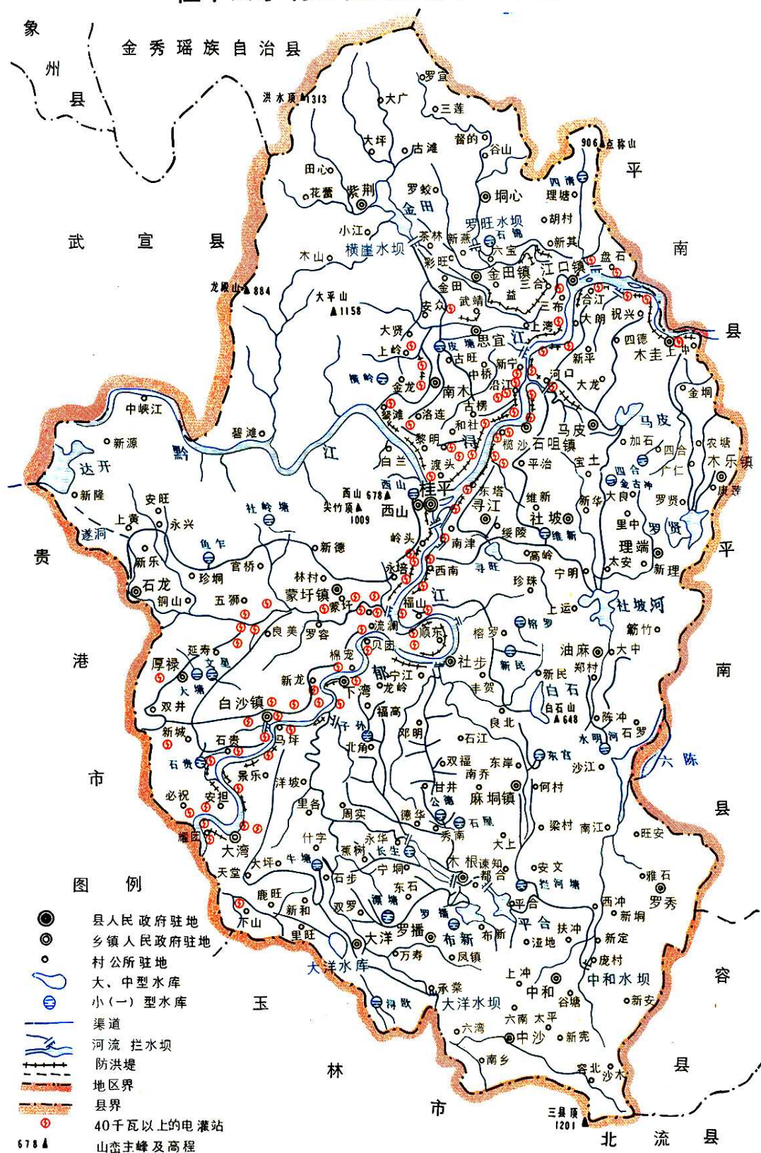
桂平县水利工程灌区现状分布图
