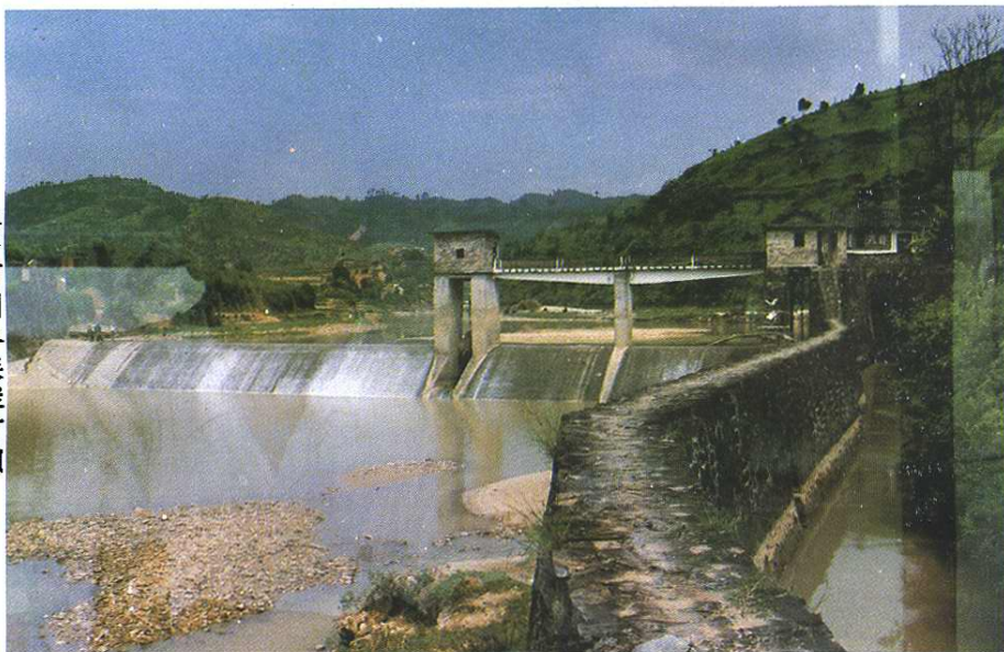
大洋河引水渠拦河坝
