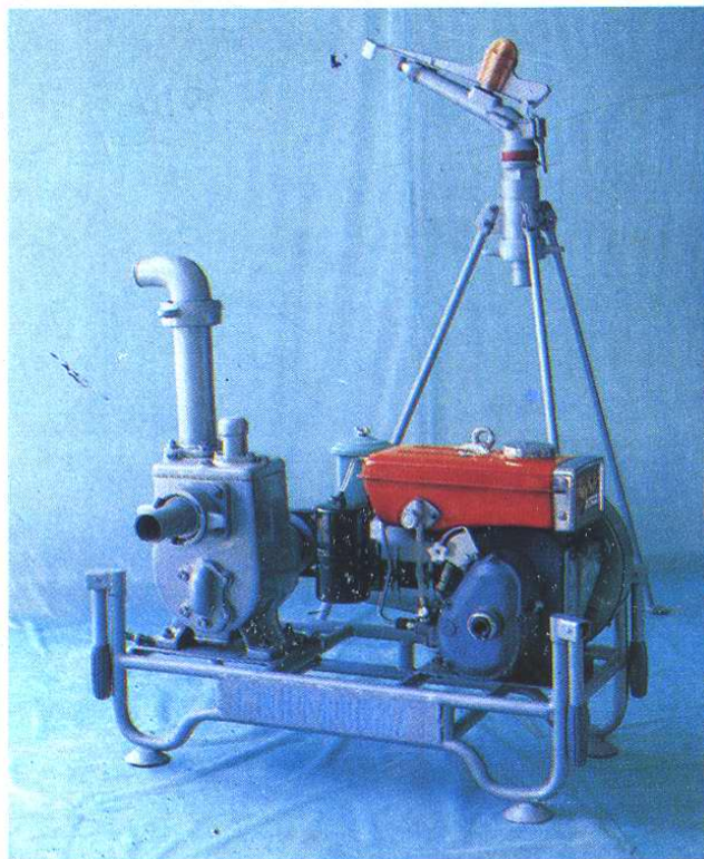
「金田」Ⅰ型喷灌机(桂平县水电设备厂生产)
