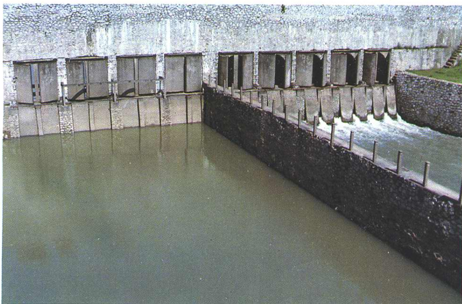
蒙圩永江防洪闸
