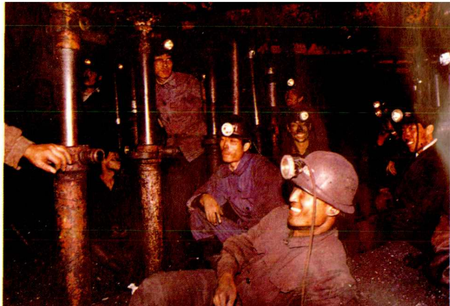
滑移支架放顶煤工作面
