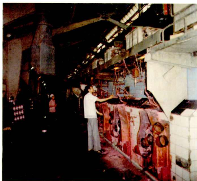
陕西兴平玻璃纤维总厂拉丝车间
