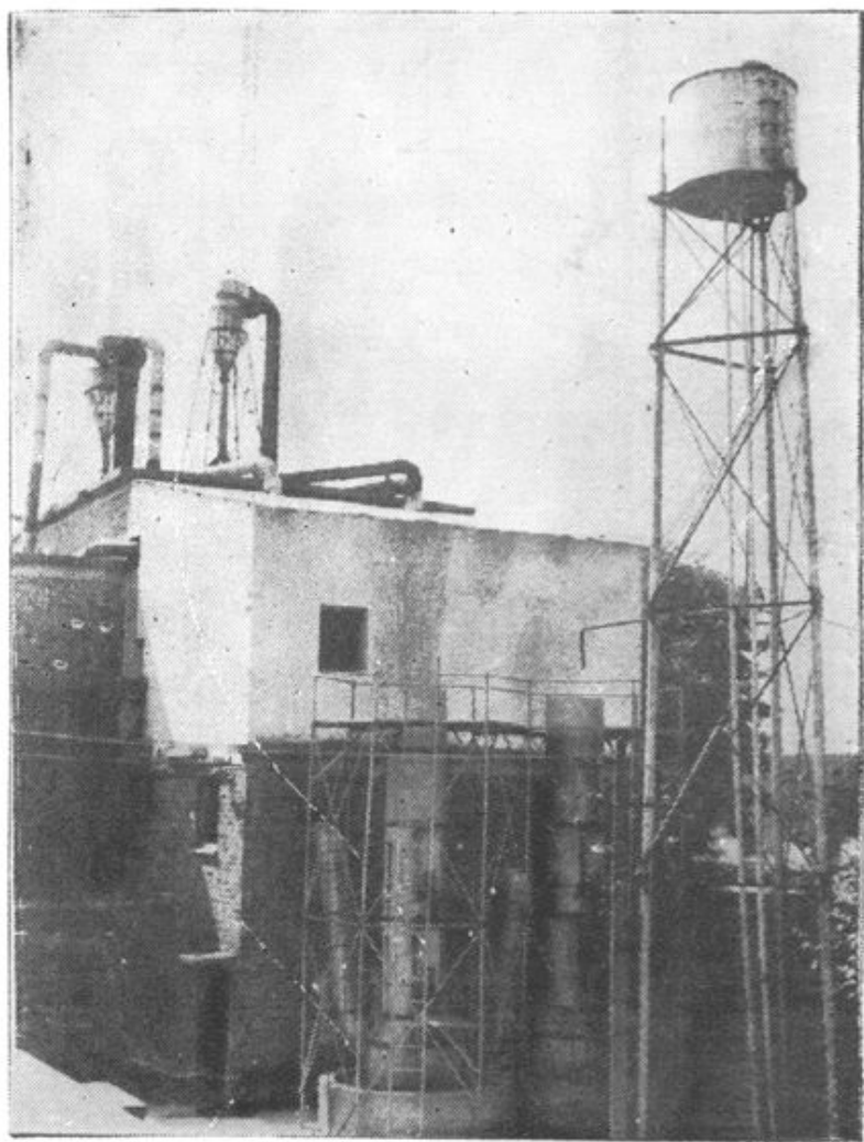
横林米厂大米车间湍流除尘塔
