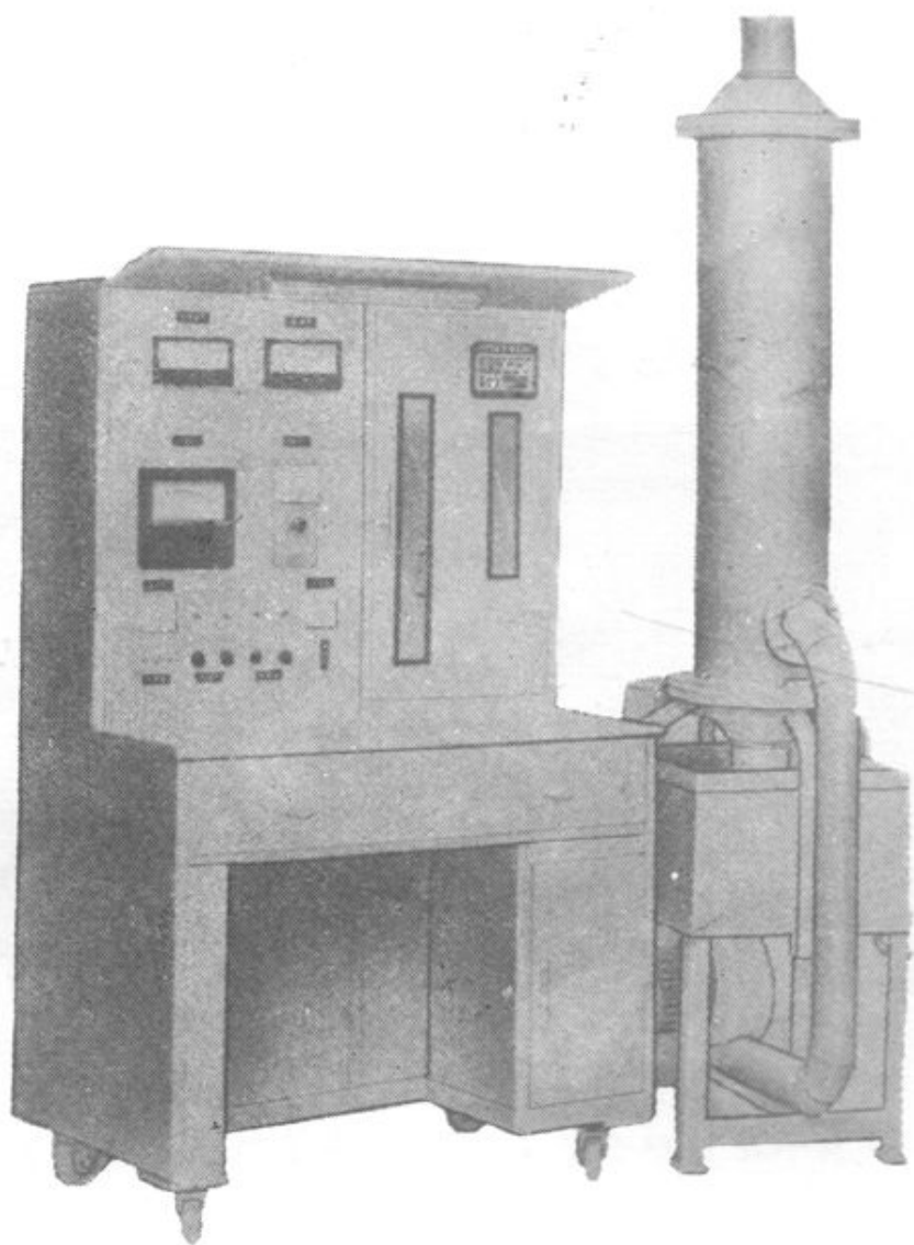
武进环保设备厂生产的动态沉积物监测器Ⅱ型
