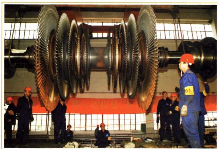
山西柳林电力有限责任公司汽轮机转子检修
