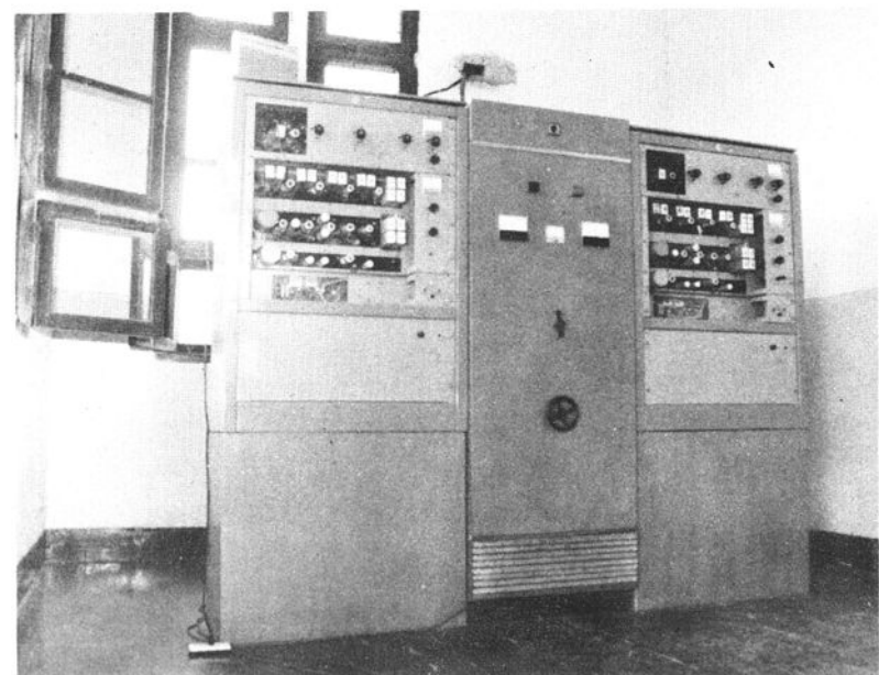
县广播站调频发射机
