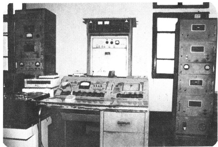
县广播站1986年10月以前主机设备
