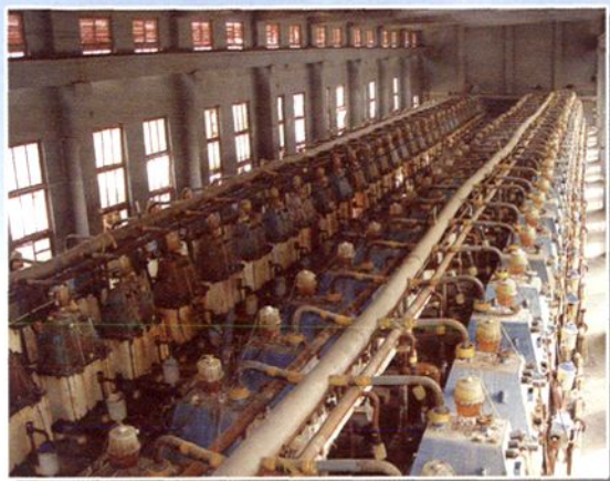
▲ 氯碱酸分厂电解槽装置
