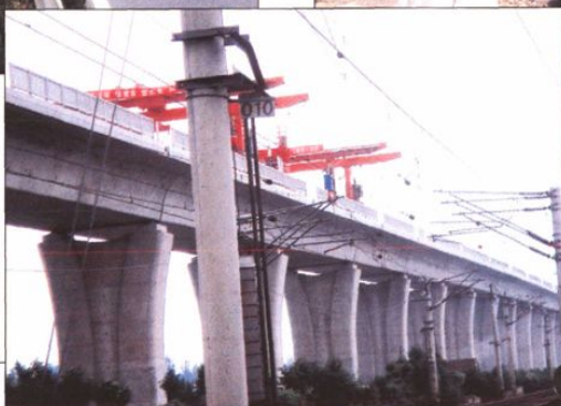
在建的沪宁城际铁路
