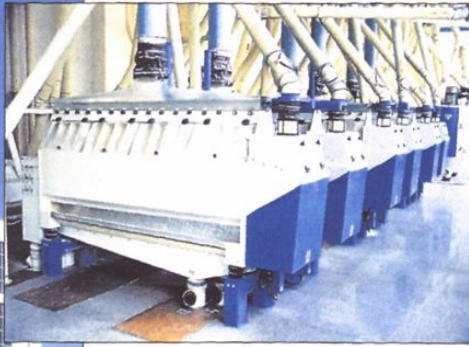
进口意大利面粉生产设备
