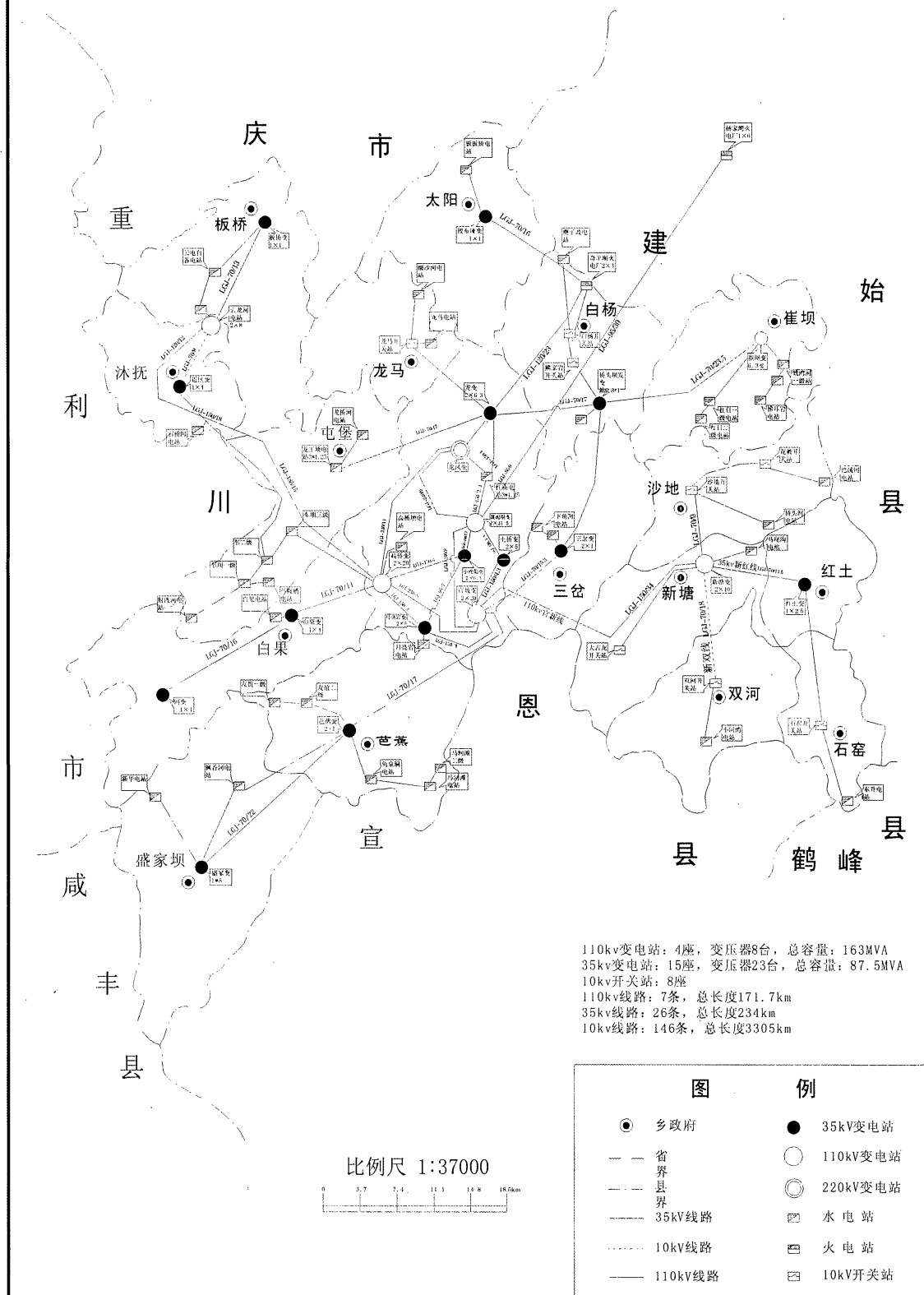
2005年恩施市电网地理接线图
