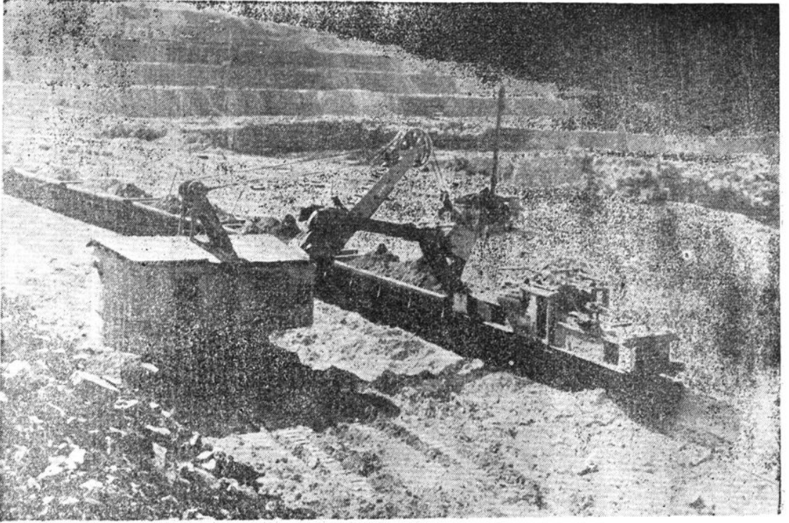
矿山北一采矿场一角
