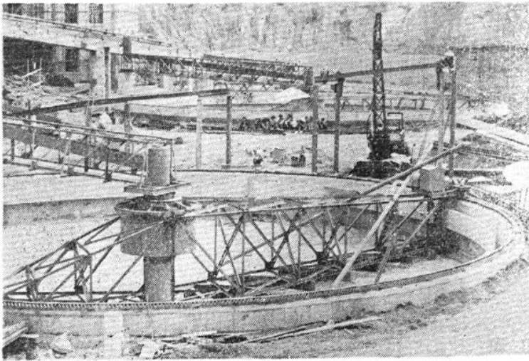
富粉溢流选矿厂一角
