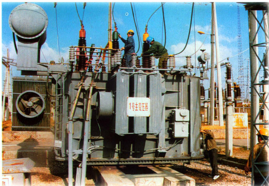
技术人员在伊宁市西郊变电所对主变压器进行维护。
