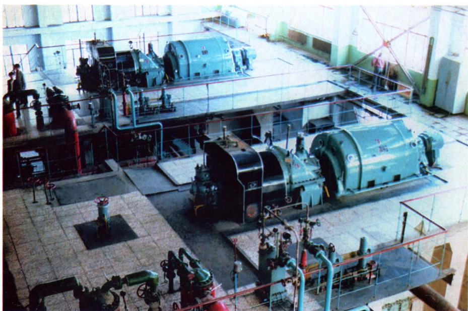
伊犁第一火电厂5号、6号机组发电车间全景。
