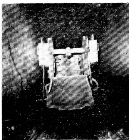
△攸县吉林桥煤矿井下正在工作的耙斗装岩机
