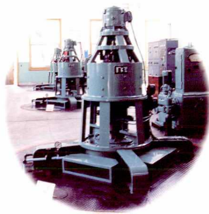
赋石水库水电站立式水轮发电机组
