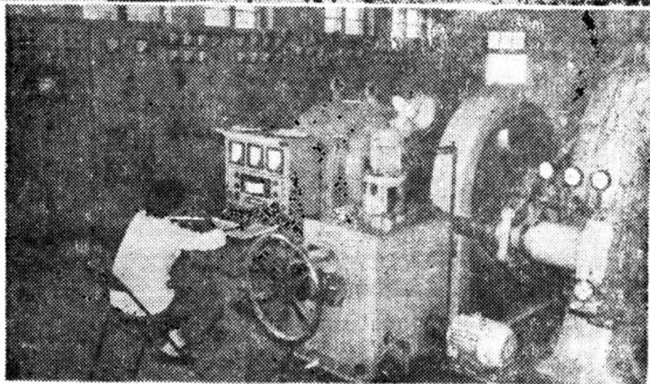
②庙尔沟东电站内景
