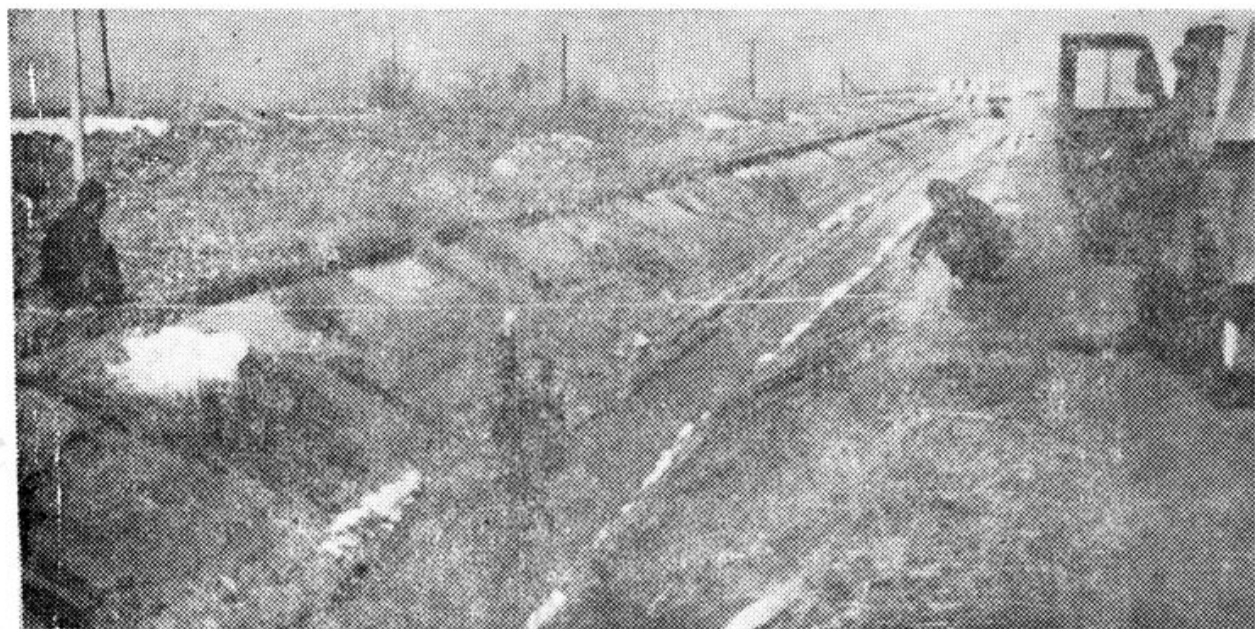
⑥管道处技术人员实测管道冻胀
