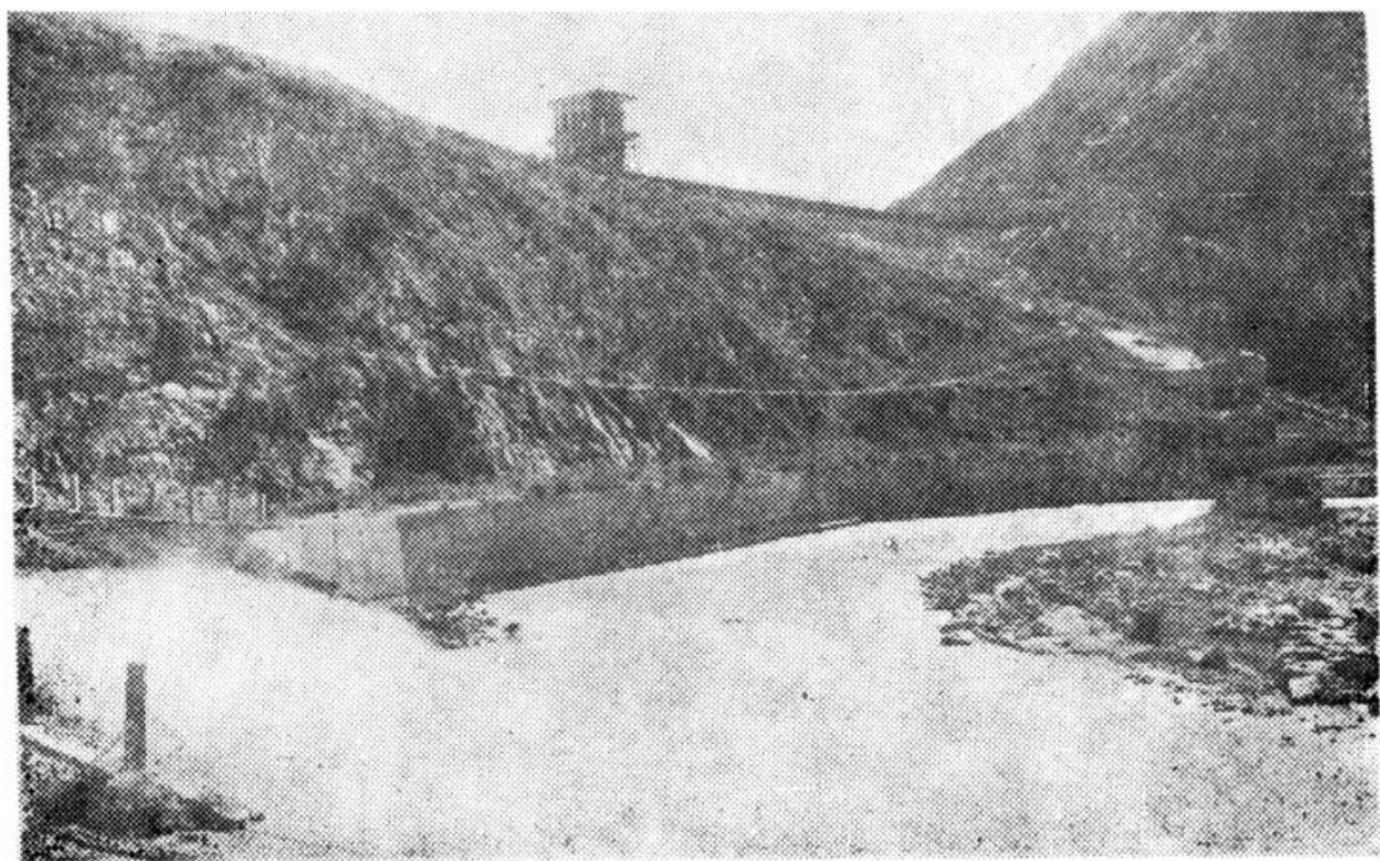
①头屯河水库大坝主体（下游）
