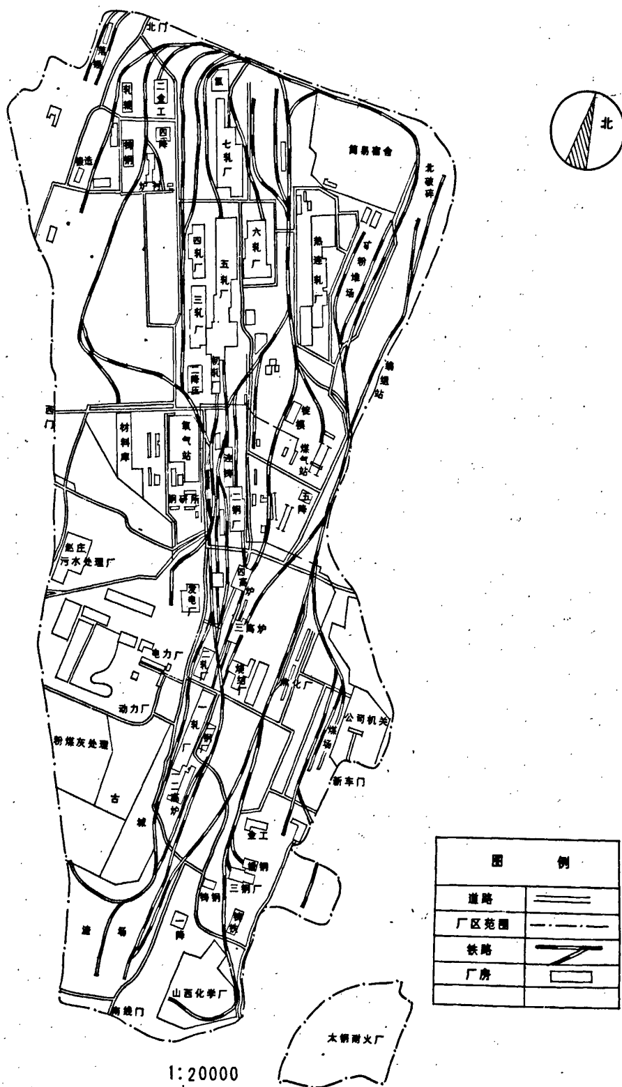
太原钢铁公司平面图(主厂区)
