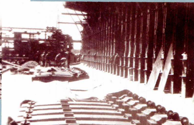
1937年9月7日 建设中的36孔焦炉
