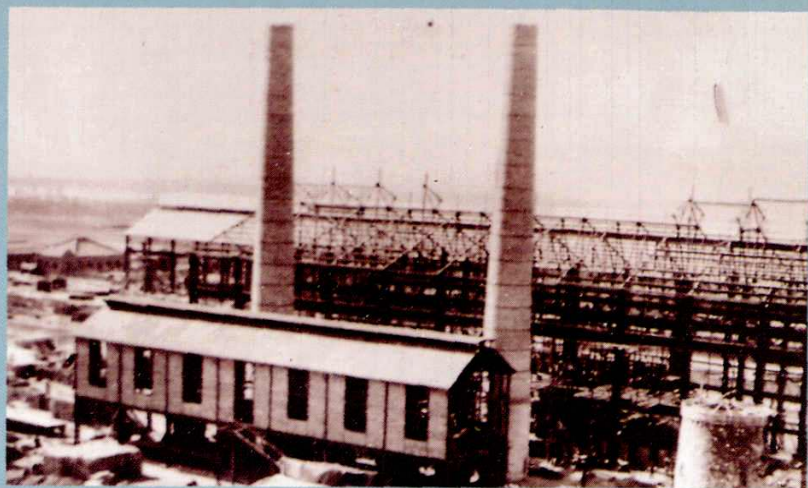
1936年10月20日建 设中的平炉炼钢车间
