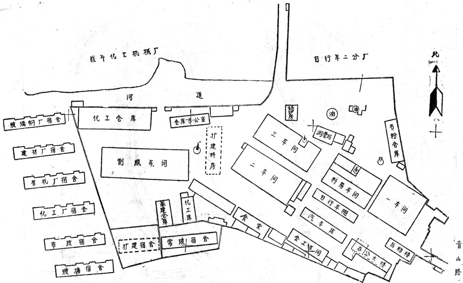
常州市玻璃厂厂区平面图
