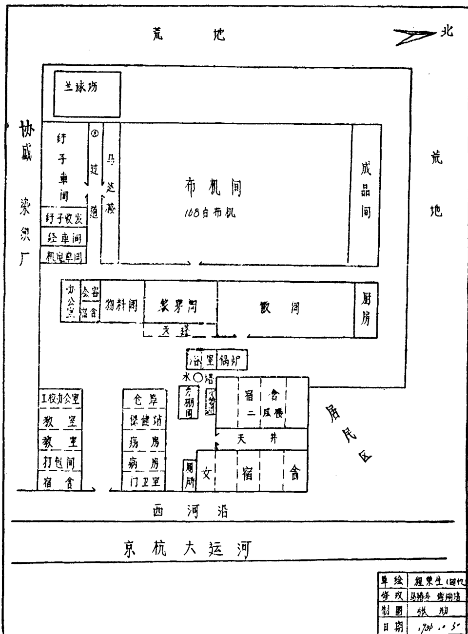
(一九五五年)并厂前协威染织厂平面图 面积4666.69M 2
