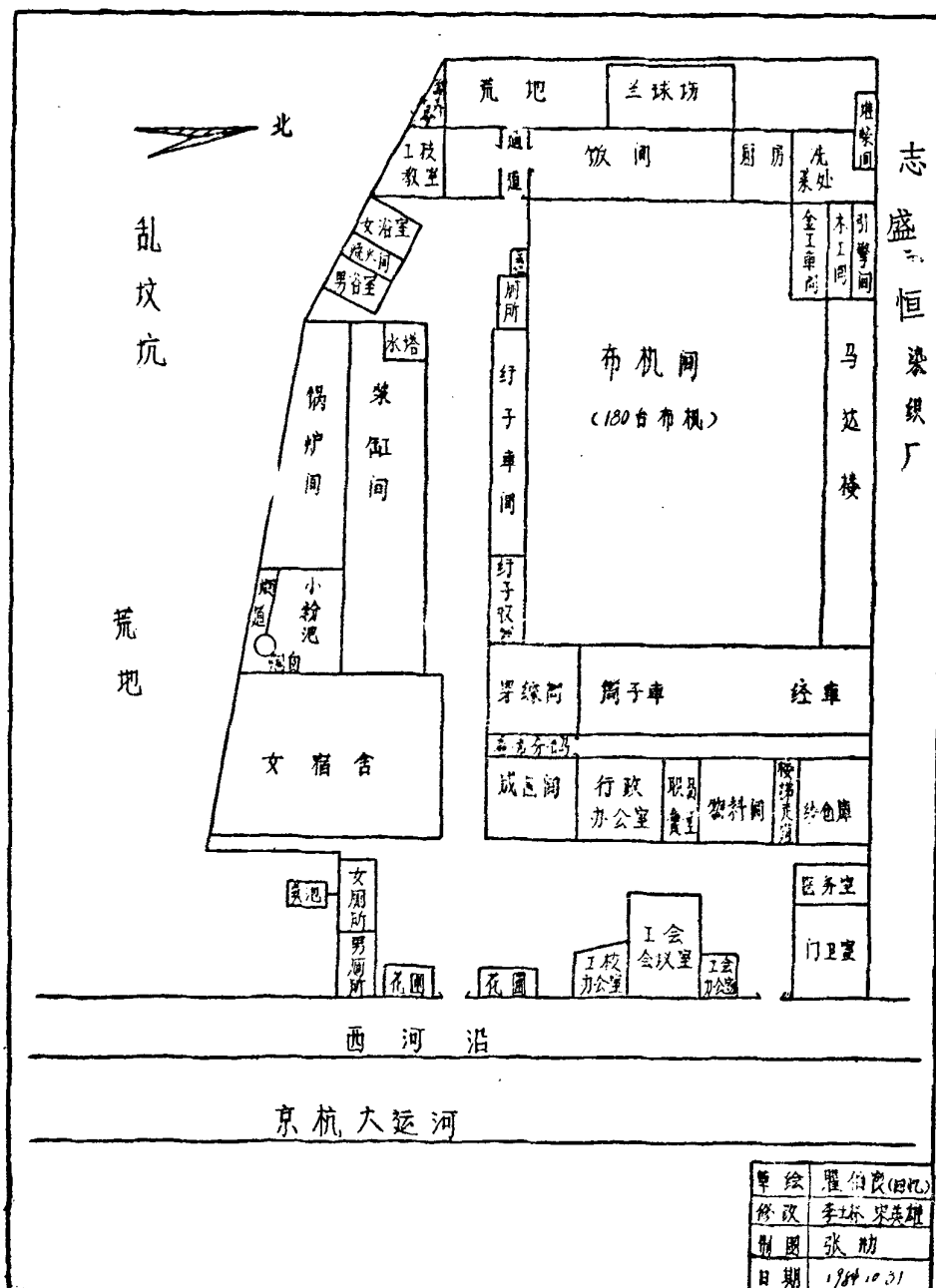
(一九五五年)并厂前志盛恒染织厂平面图 面积6000M 2
