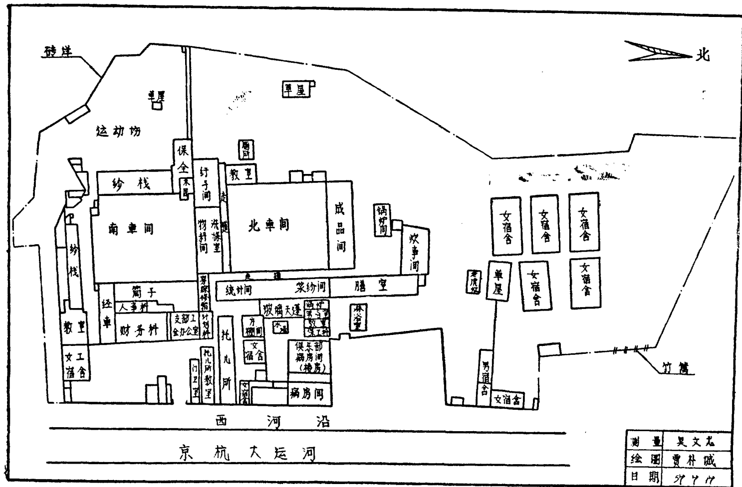
公私合营协成染织厂全厂平面图 总面积约22904.743M 2
