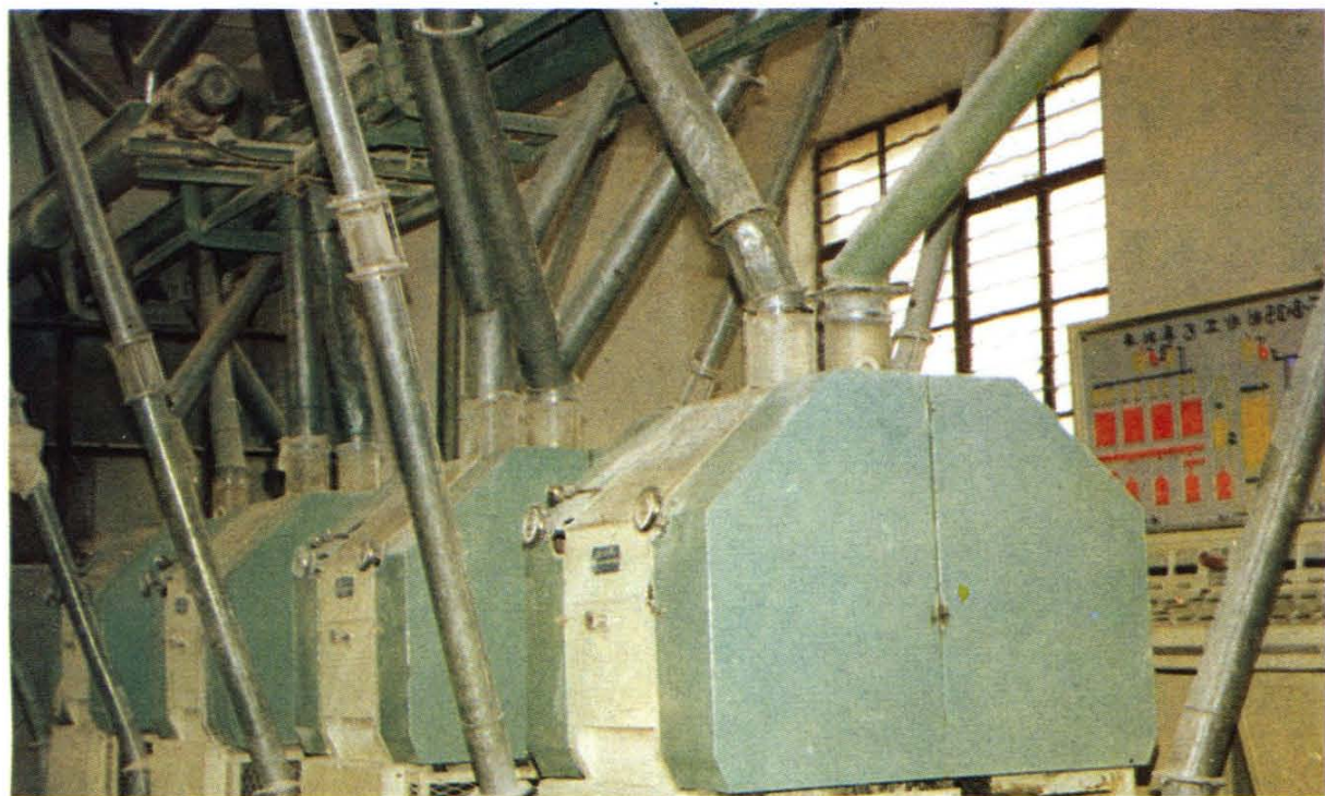
日产 500 袋 FM35 型磨面机
