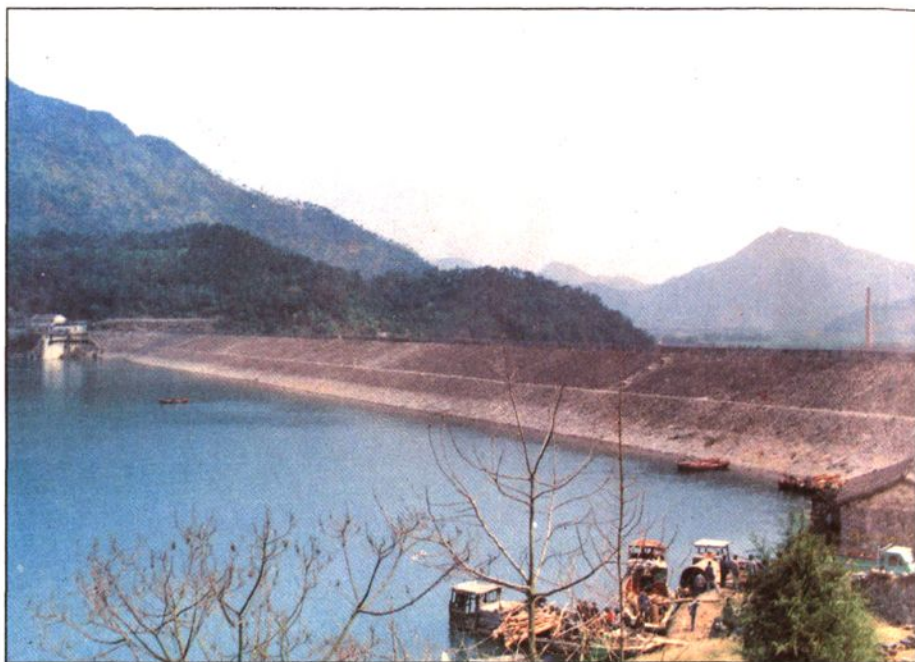
这是1958年10月至1964年底的六年期间，由国家财政投资 2837.17 万元兴建的黄岩最大的水利工程——长潭水库，它的大坝高度为35.5米，最大库容为6.91亿立方米，使黄岩、温岭、椒江和临海西岑乡的100多万亩农田受益。
