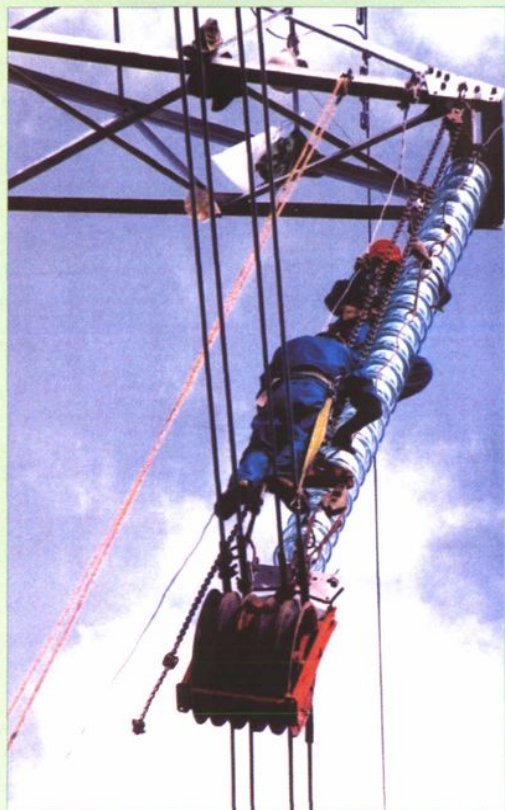
达(拉特电厂)包 (头高新变电站)500 千 伏输电线路在进行附件 安装(2003)
