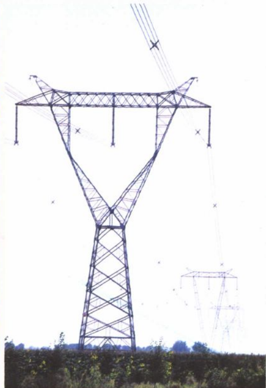
准(格尔电厂)永(圣域变电站) 500 千伏输电线路之一段(2001)
