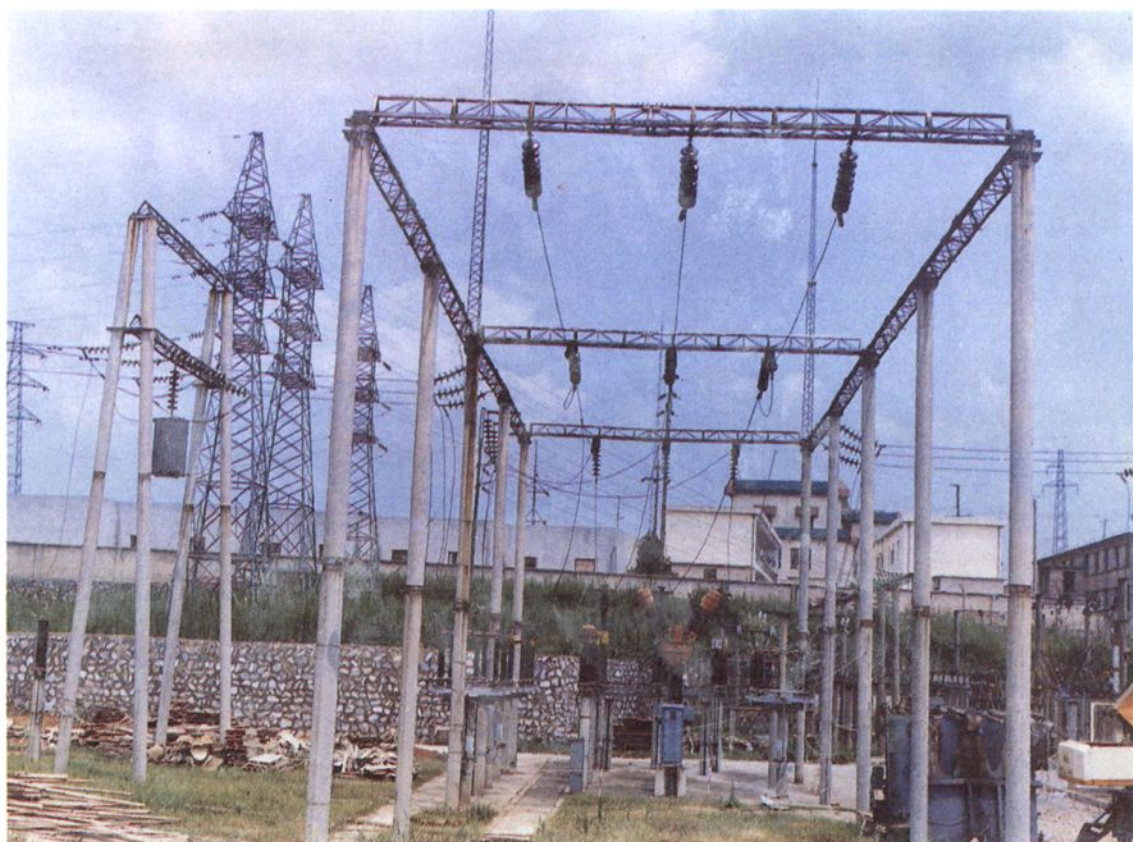
▲县变电所一角
