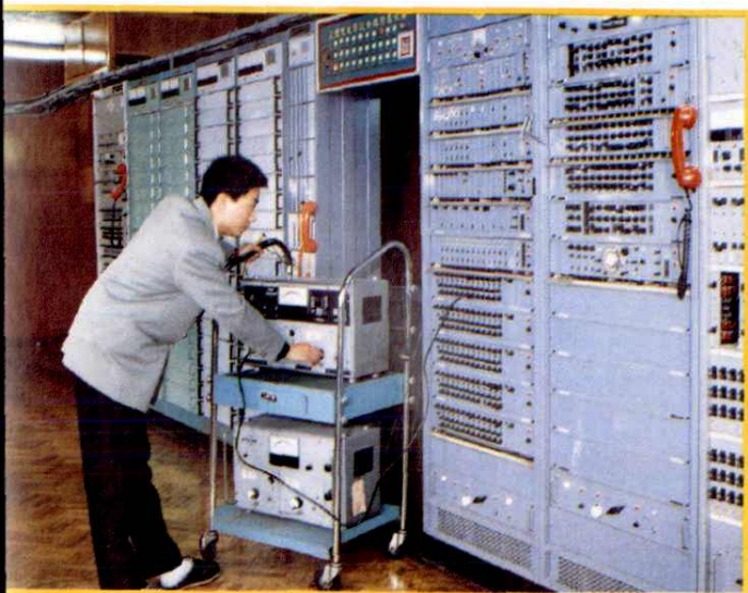
衢州电力局调度所微波通信机房
