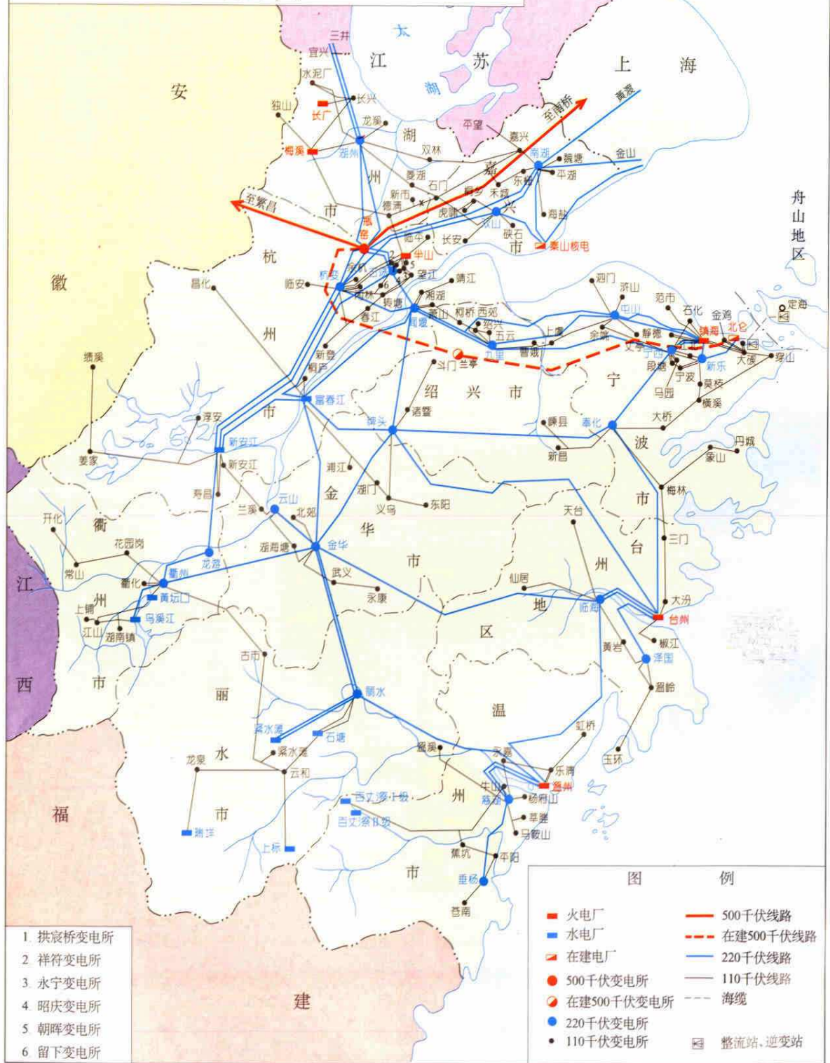
浙江省110千伏及以上电网地理接线示意图 (1990年)
