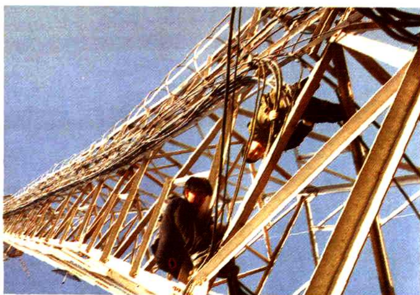
2001年1月移动分公司机务员在安装那林套海基站
