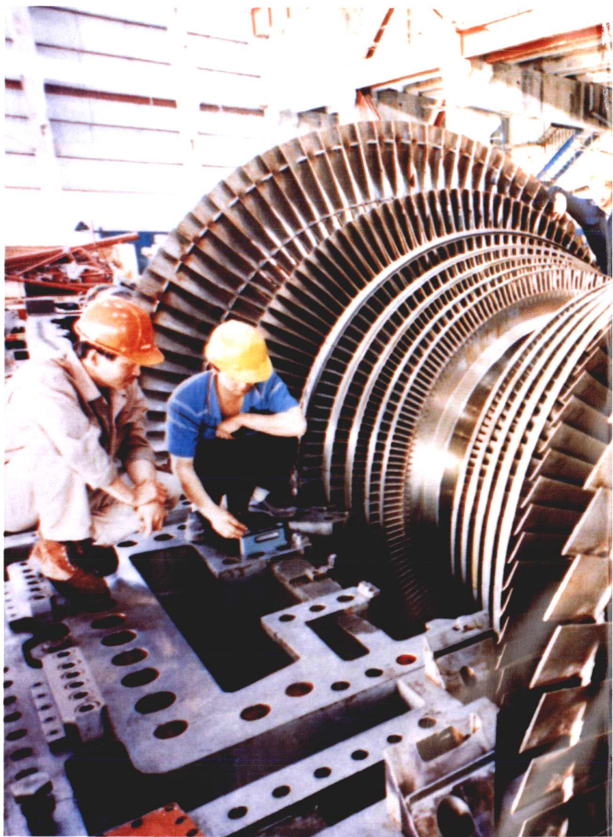
北仑电厂 60 万千瓦汽轮机安装
