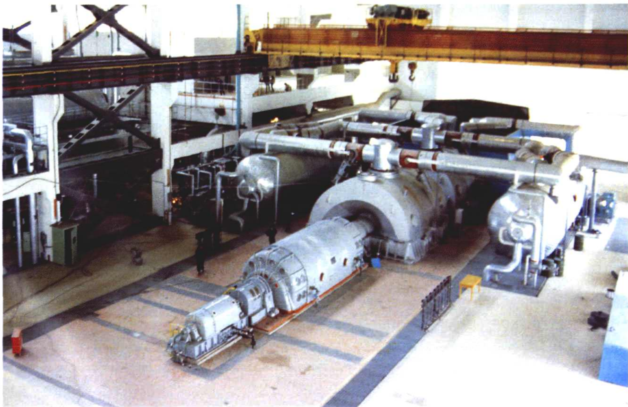
秦山核电厂 30 万千瓦汽轮发电机组
