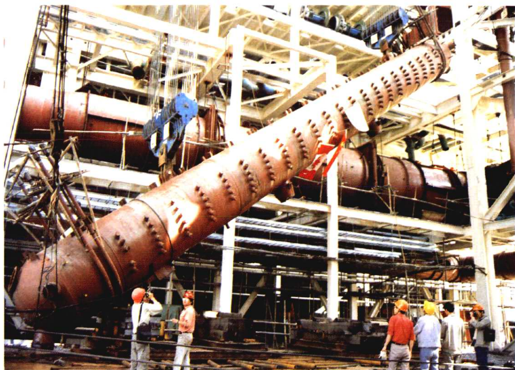
北仑电厂 60 万千瓦发电机组锅炉汽包吊装
