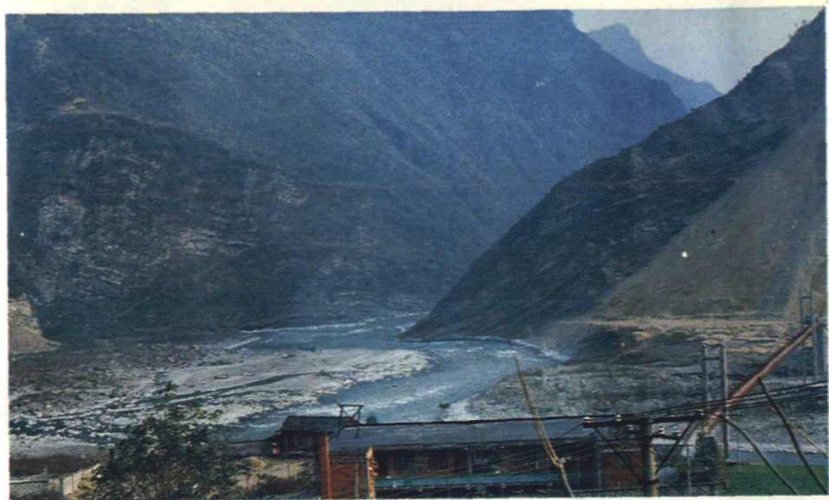
▲ 通口河袭夺湔江的袭湾——北川县银屏口。
