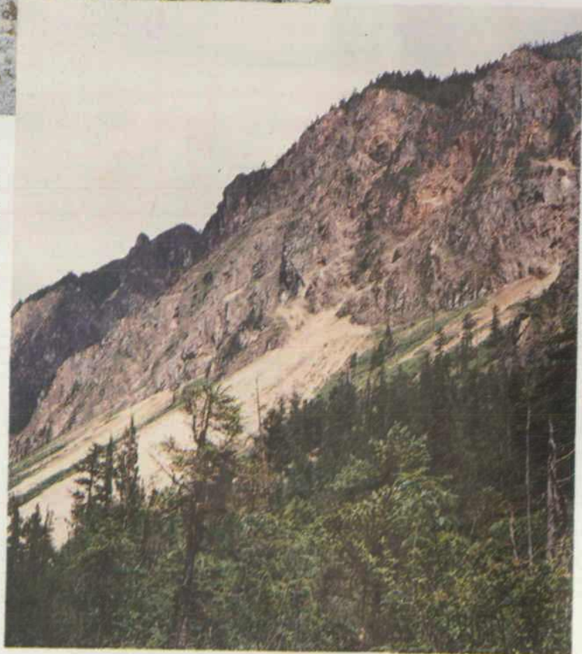
平武县王朗自然保护区竹根岔西坡的山地滑坡。
