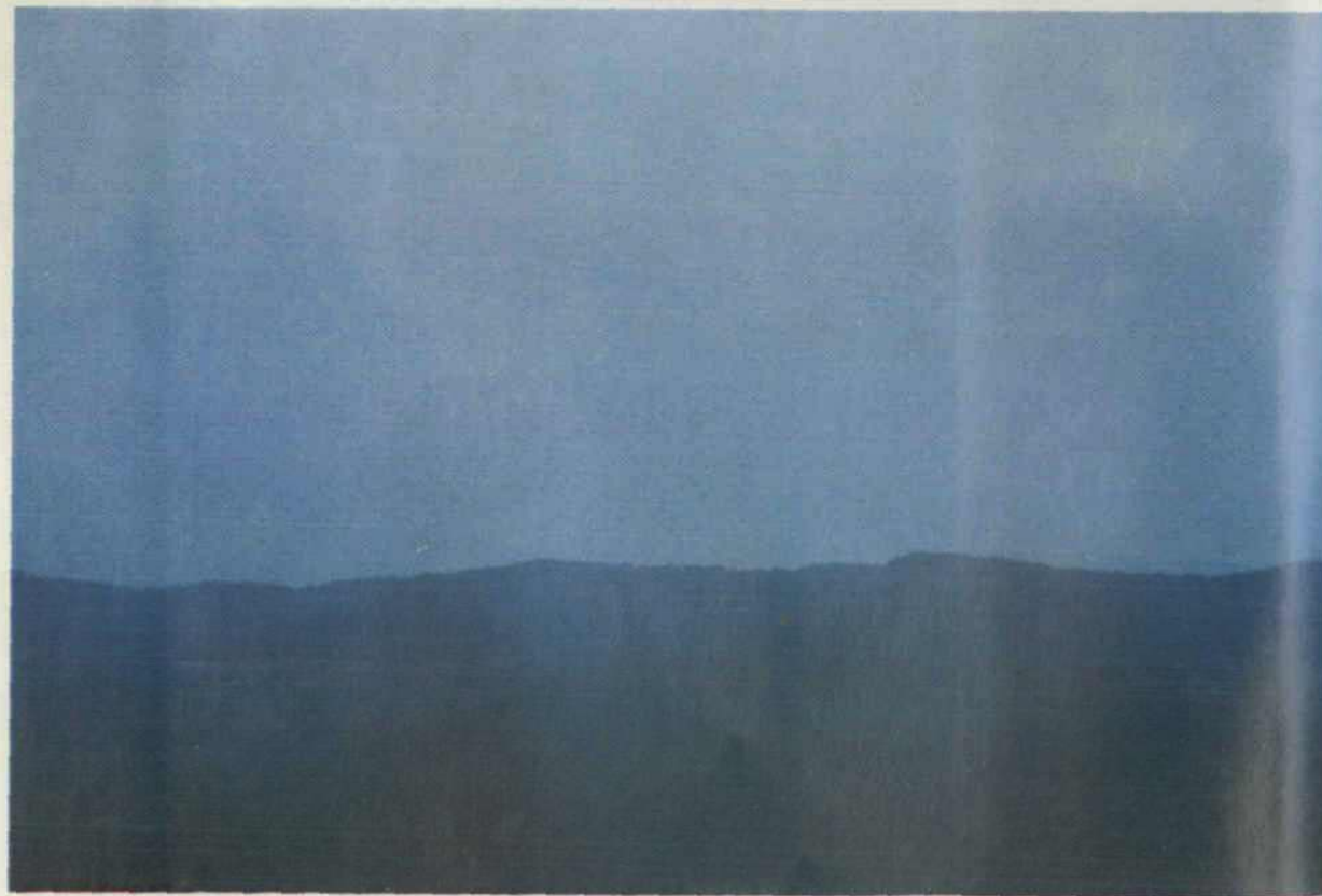
▼ 第三纪末七曲山期（剑门期）梓潼县七曲山东面之夷平面带。
