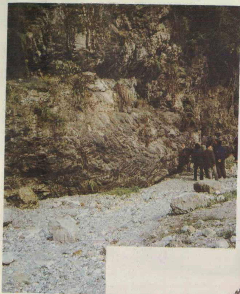
平武县两河堡公路侧发育在志留系茂县群的小褶皱构造。
