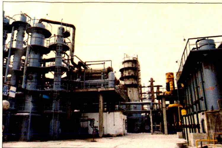
▲ 酮苯脱蜡 (油)装置
