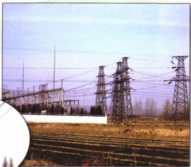
220千伏输电线路
