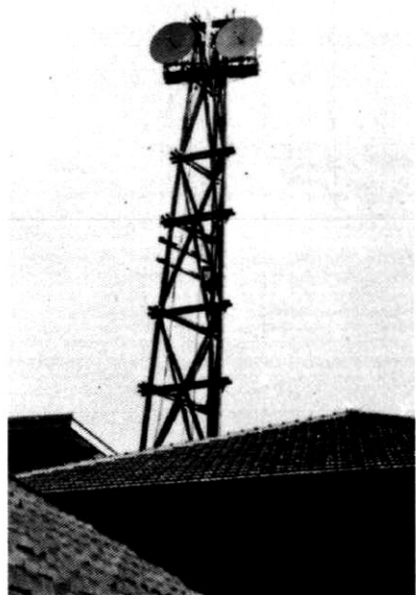
▲六十年代的木质微波塔。
