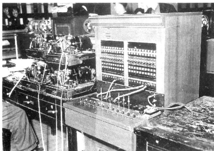
▲1959年,长沙市电信职工自制的电报交换机。
