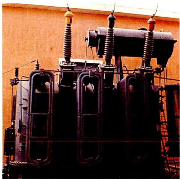
金桥站 110/35 千伏 6.3 万千伏·安 2 号主变压器
