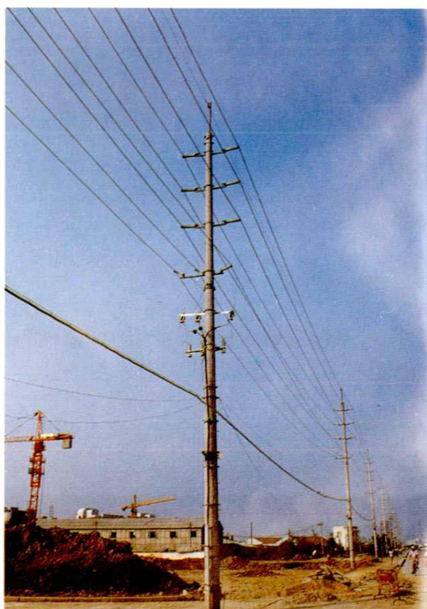
35 千伏单杆双回路线路
