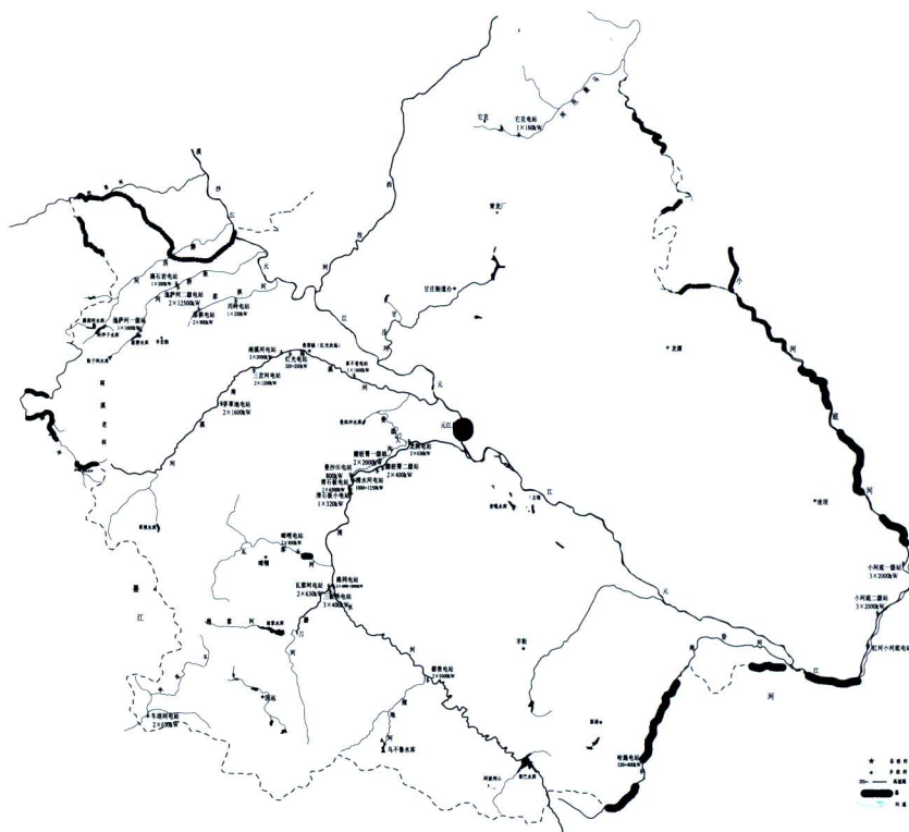
元江县小水电站分布图
