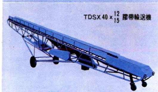
东海县粮食机械厂胶带输送机
