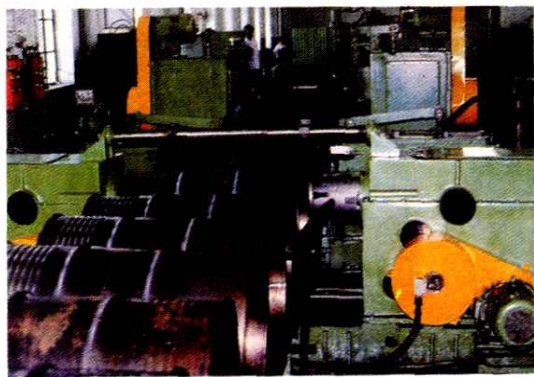
东海县粮食机械厂钢油桶生产流水线
