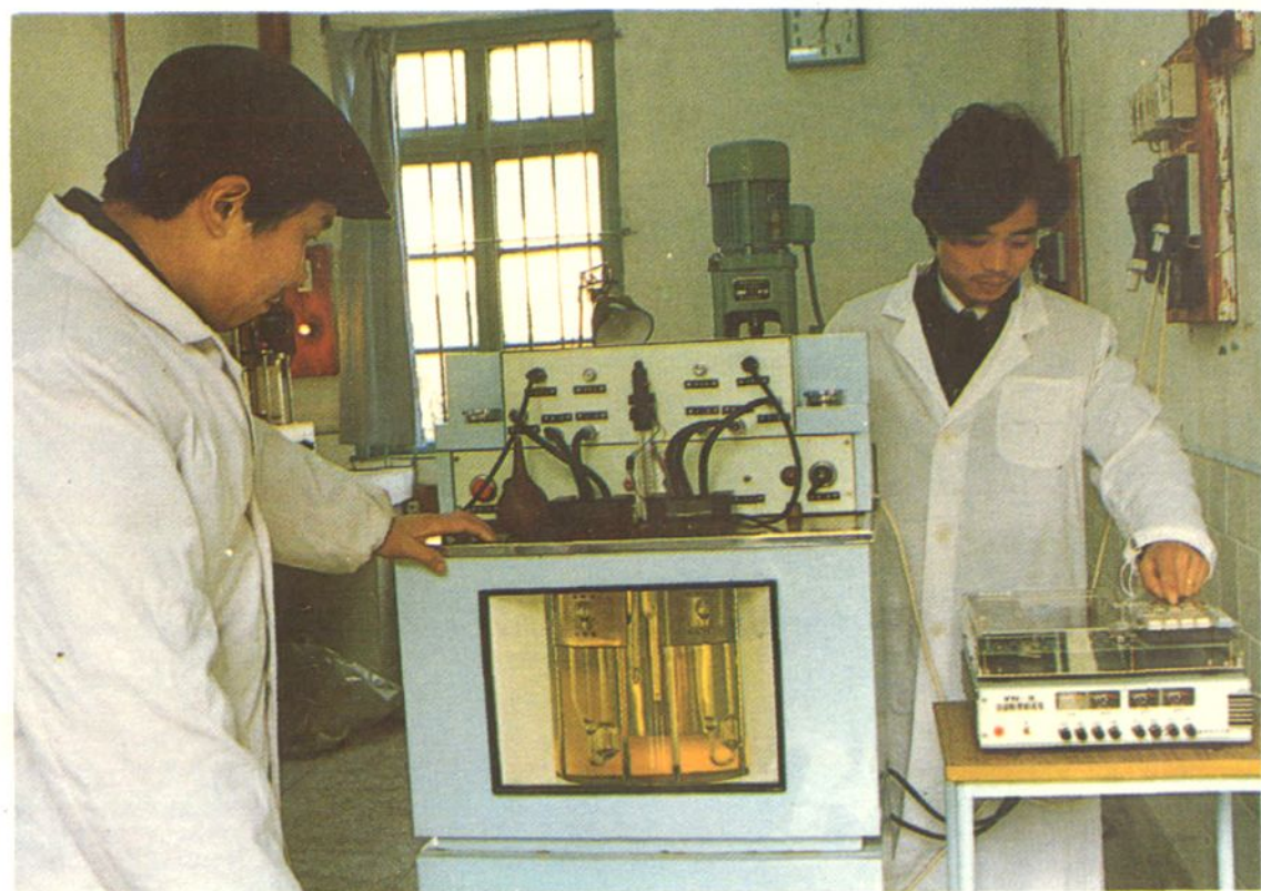
杭州小河油库化验室在做油品试验
