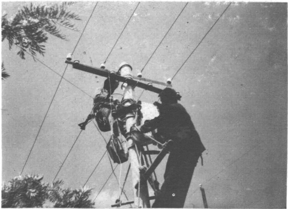
架设输电线路
