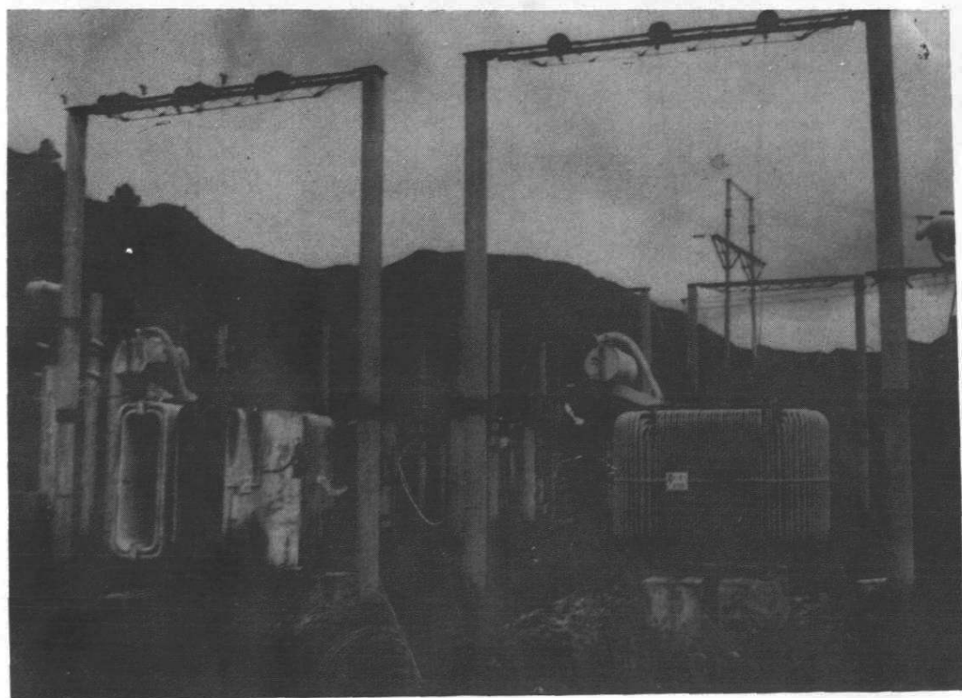
马鞍电站( 3 \times 1600 千瓦)变电站
