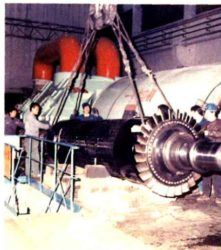
▲发电机转子吊装
