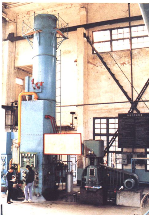
▲140/660-1 制氧分馏塔
