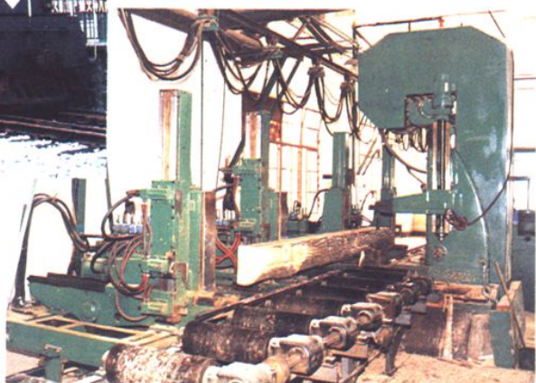
▲MJ3212 带锯机
