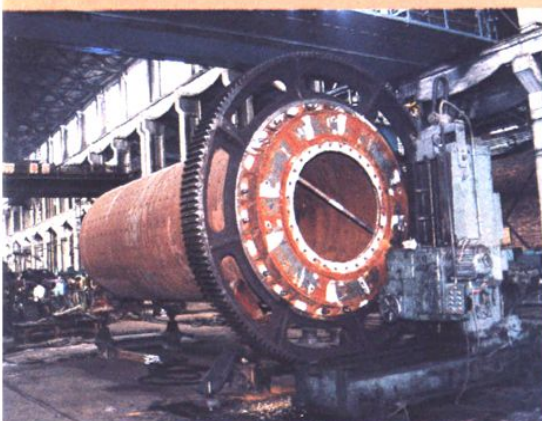
▲球 磨 机
