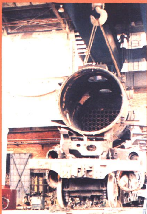
▲100吨 天 车
