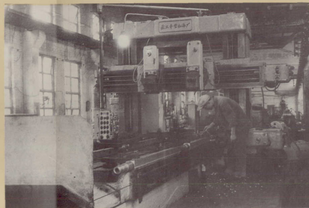
龙门刨
