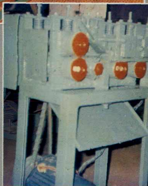
开片滚平机
