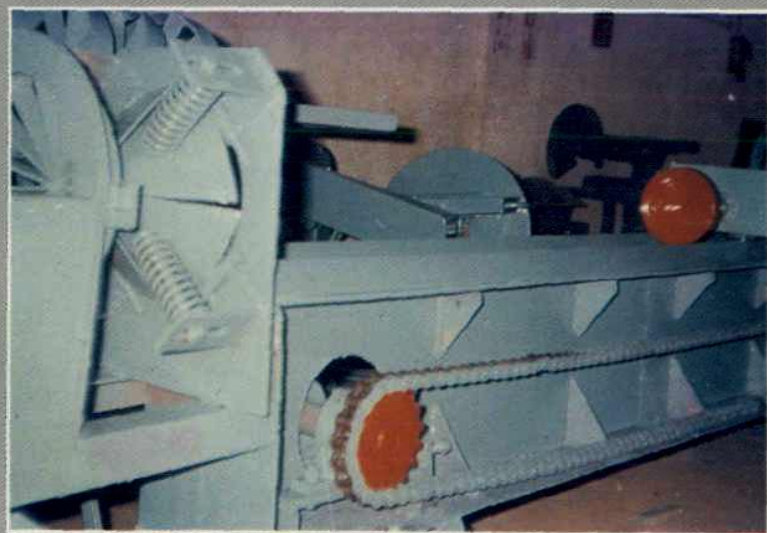
大型破竹机
