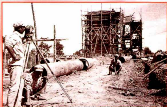
筹建勘测
