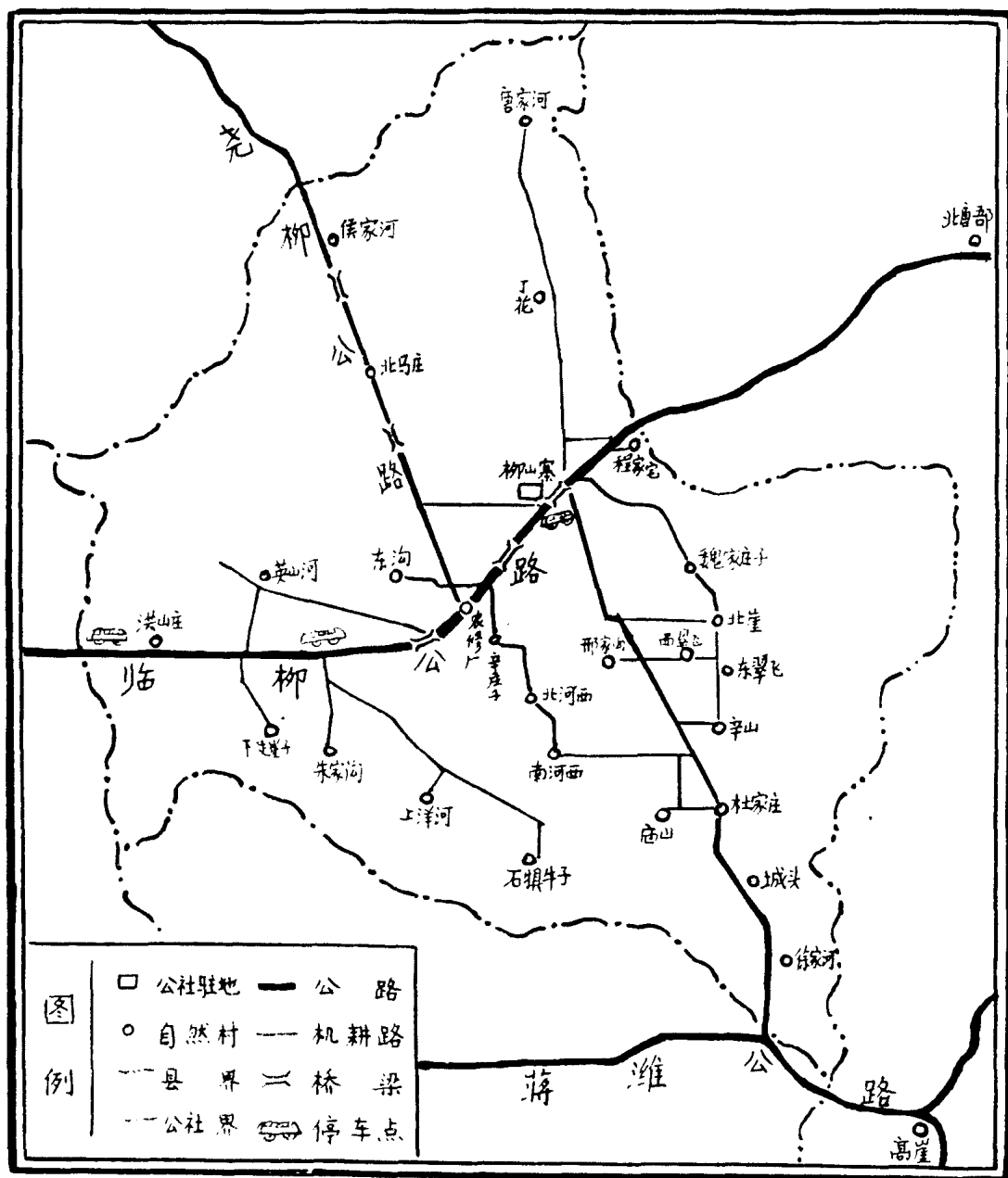
柳山公社交通现状图
