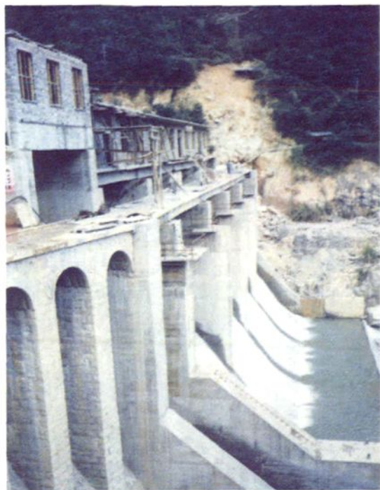
16 南靖船场溪三级电站装机容量 8000 千瓦
