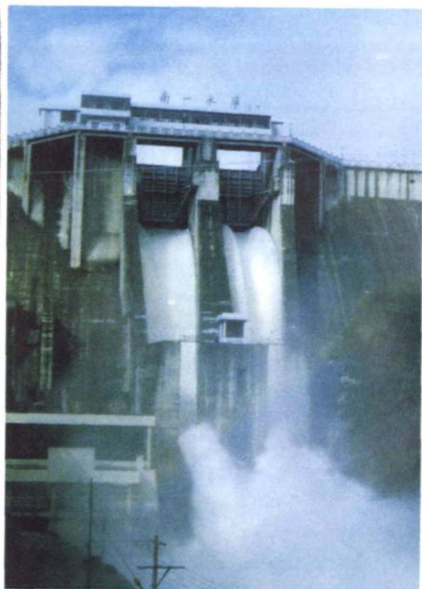
15 南靖船场溪一级 电站装机容量 2 万千瓦
