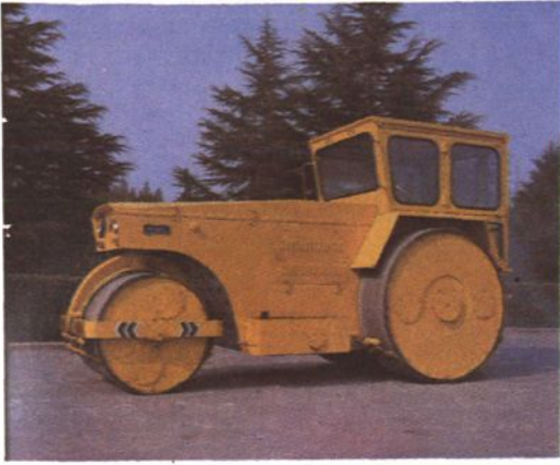
“部优产品”3Y 12/15 压路机
