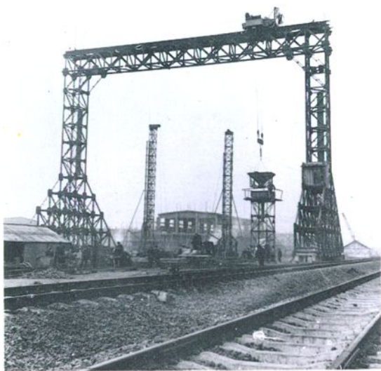
自制万能杆件组装架桥机
