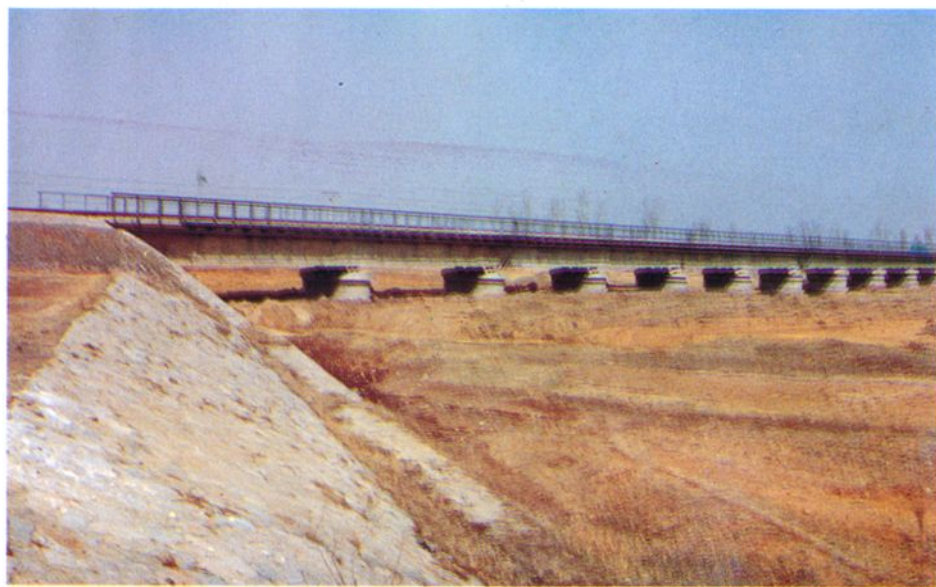
兖州矿区白马河铁路大桥全景
